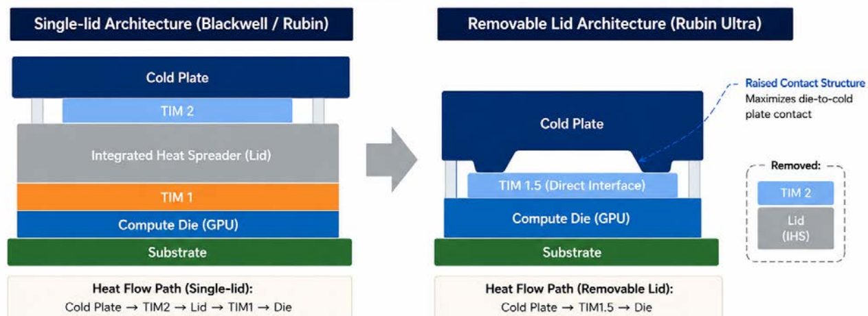
圖 5：Rubin Ultra GPU 世代預計採用可拆卸式上蓋設計，帶動 ASP 持續提升
